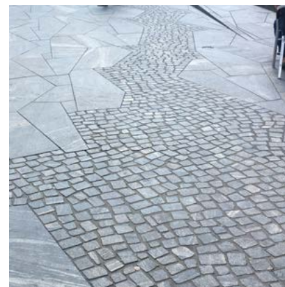
VER 3: Erikoislaatta, suunnaton mosaiikkinen ladonta Variaatio pintakäsittelyllä tai yhdistämällä peruskiveen kuten nupu- tai noppakivi.
