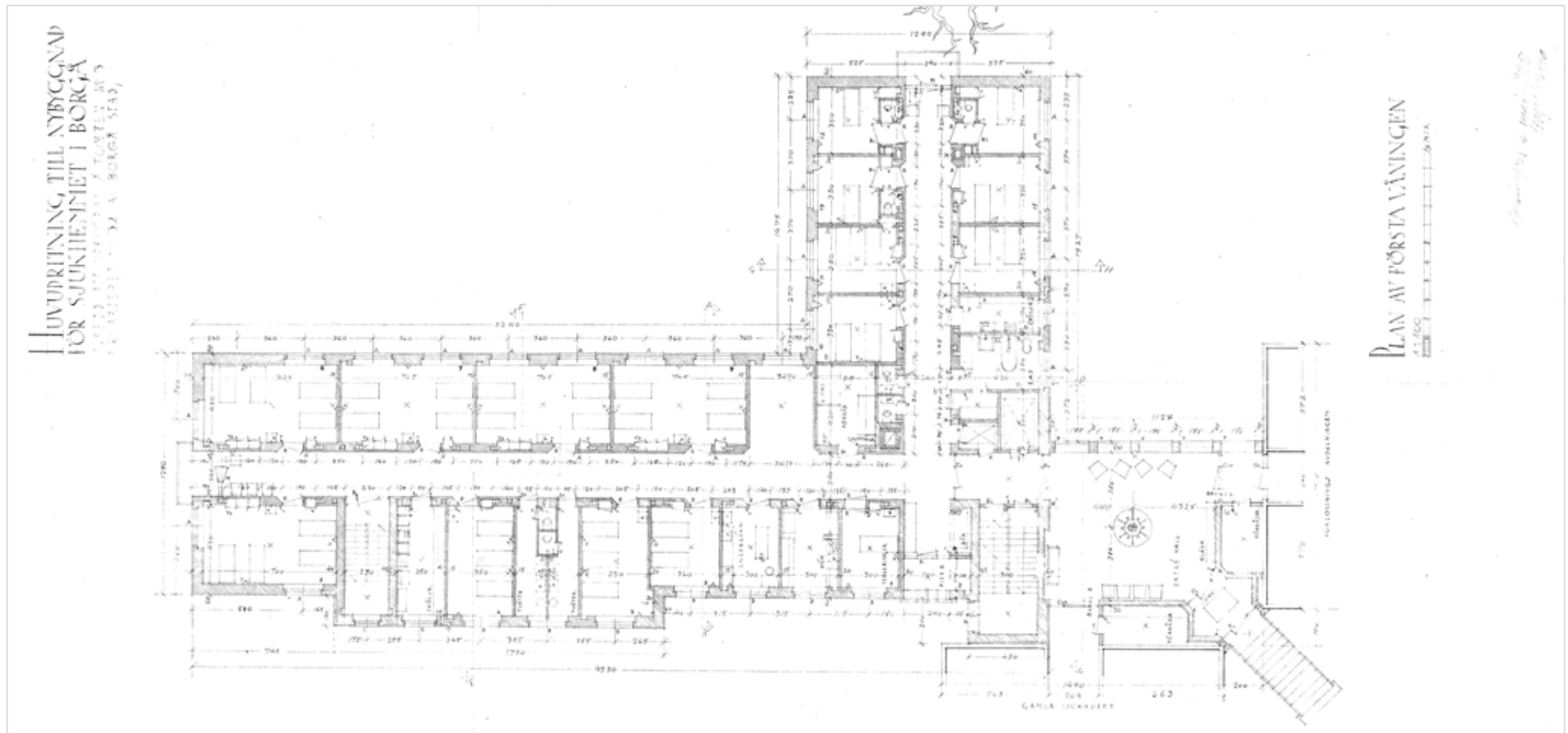
↑ Rakennuksen ensimmäinen kerros. Kerroksessa sijaitsi sisäänkäyntiaula, potilashuoneet ja toimenpidetilat. Pääpiirustus, Uno Ullberg, 1938. Porvoon rakennusvalvonnan arkisto.
