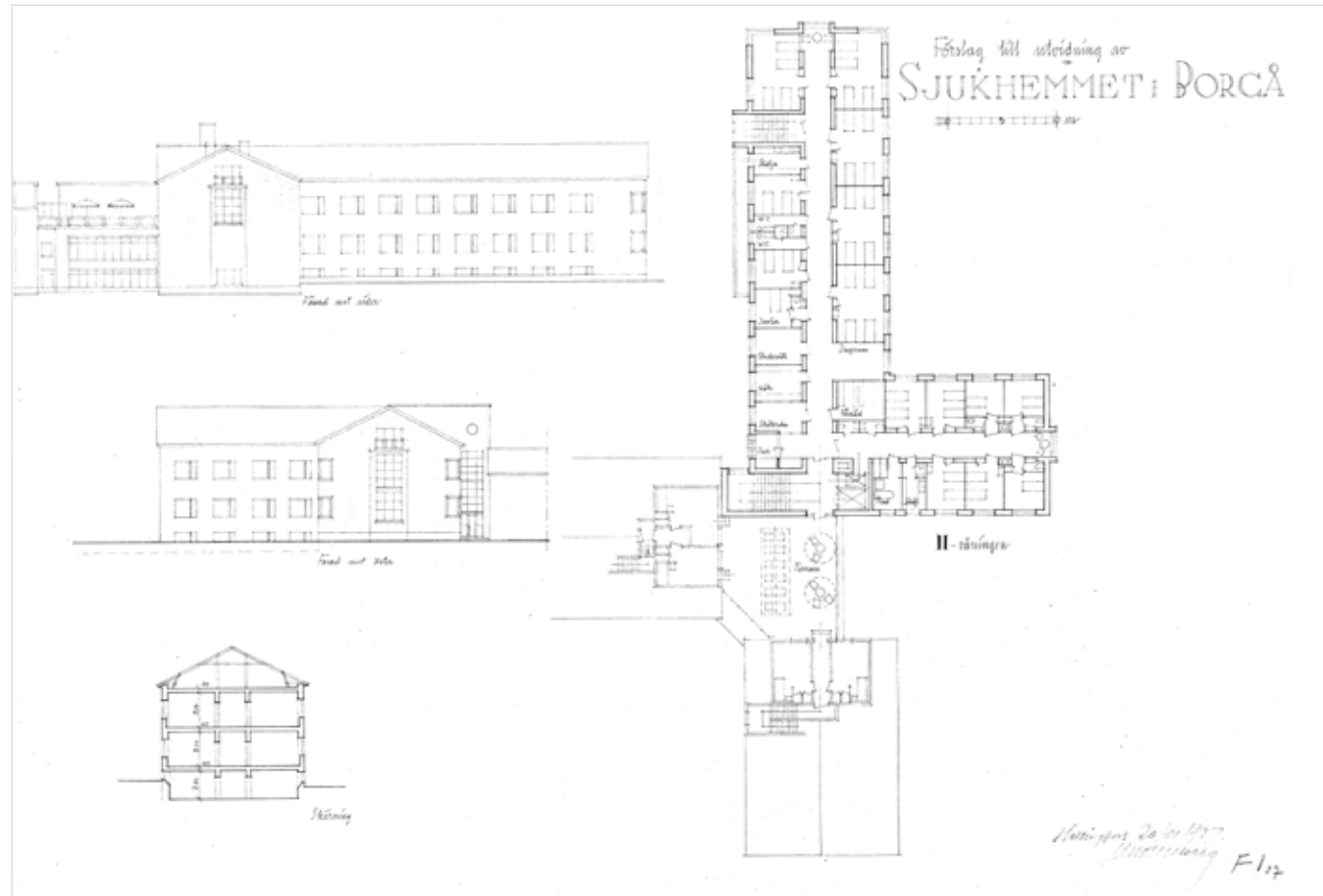
↑ Sairaalarakennuksen toinen vaihtoehto. Rakennuksessa olisi ollut yksi kerros enemmän eli kaksi potilashuonekerrosta. Muuten ratkaisu oli lähes toteutuneen vaihtoehdon mukainen. Uno Ullberg. Porvoon rakennusvalvonnan arkisto.
