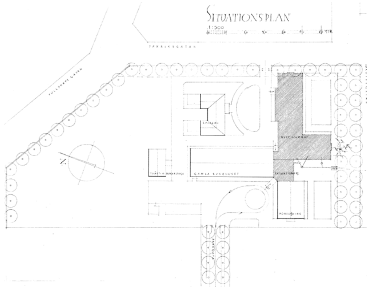
↑ Asemapiirros vuodelta 1938. Huomaa pohjoisnuoli. Uusi, vanhojen rakennusten väliin sijoittuva kivisairaala on esitetty tummennettuna. Pääpiirustus, Uno Ullberg, 1938. Porvoon rakennusvalvonnan arkisto.
