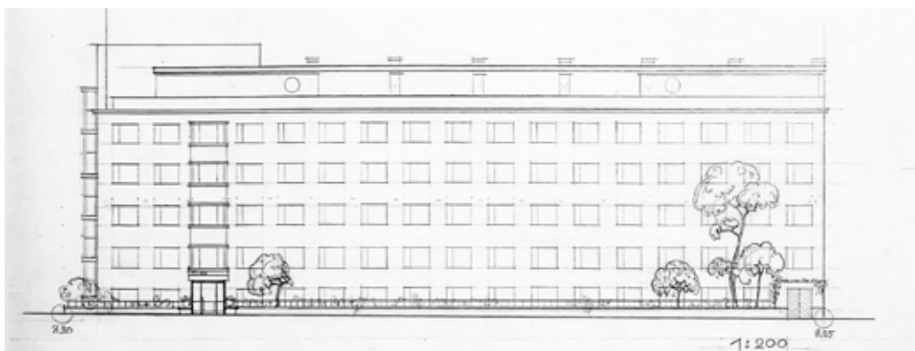
← Eiran yksityissairaalan toinen vaihtoehto eli uudisrakennussuunnitelma vuodelta 1937. Uusi sairaalarekennus olisi korvannut Sonckin sairaalan ja muodostanut tontille viisikerroksisen blokkisairaalan. Arkkitehtuurimuseo.
