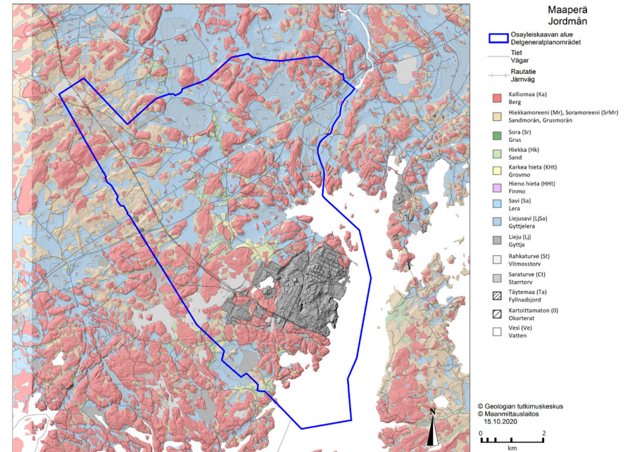
Kuva 4. Maaperäkarta.
