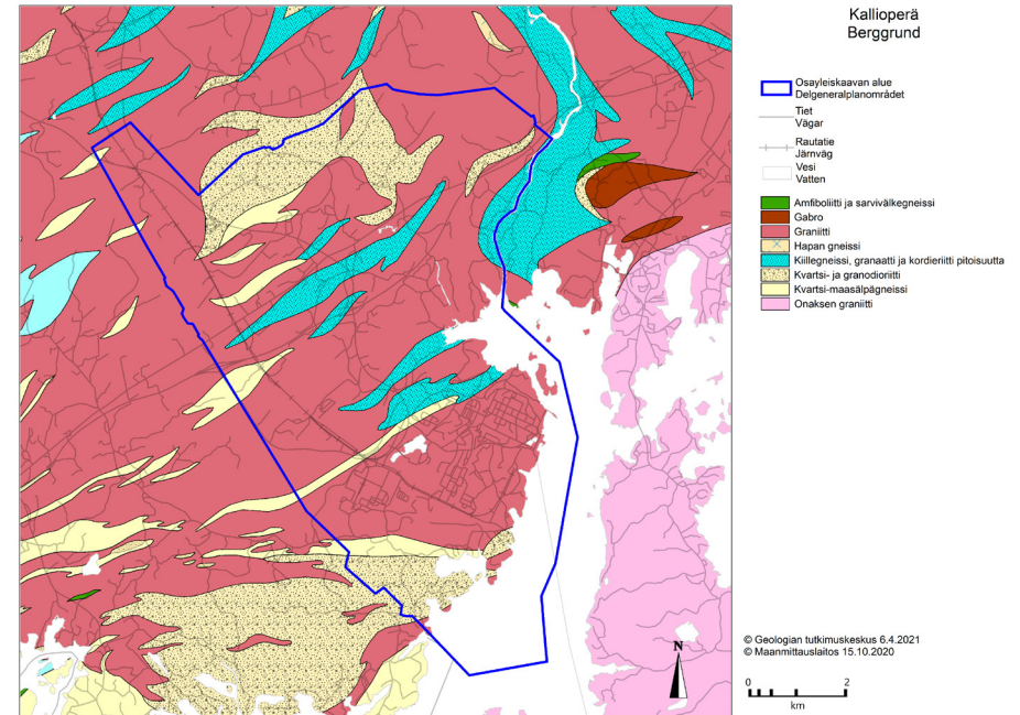
Kuva 3. Kallioperäkarta.
