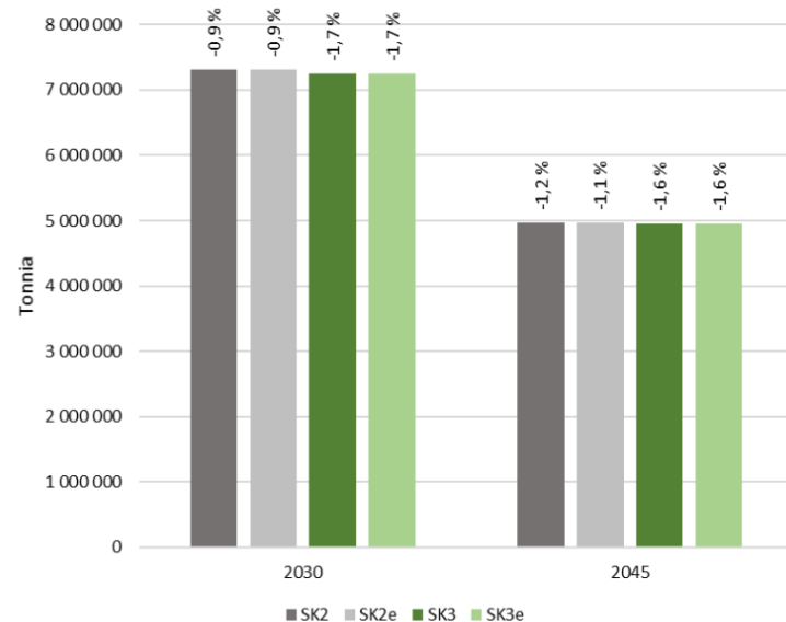
Kuva 4-10. Tieliikenteen CO 2 -päästö määrä (tonnia) ja suhteellinen muutos perussennusteseen verrattuna eri skenaarioissa vuosina 2030 ja 2045.
