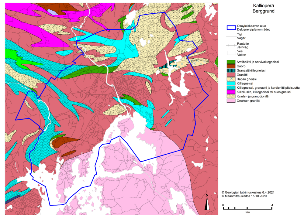
Kuva 2: Kallioperäkartta.
