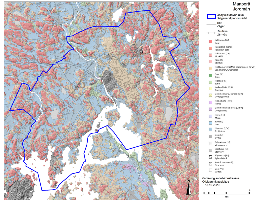
Kuva 3: Maaperäkartta.
