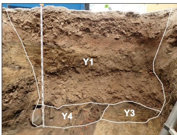
Vasemmalla: Koekuopan 3 koillisleikkaus. Oikealla: luoteisleikkaus.
