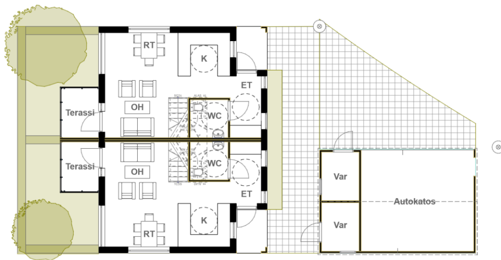
1. krs pohjapiirros
