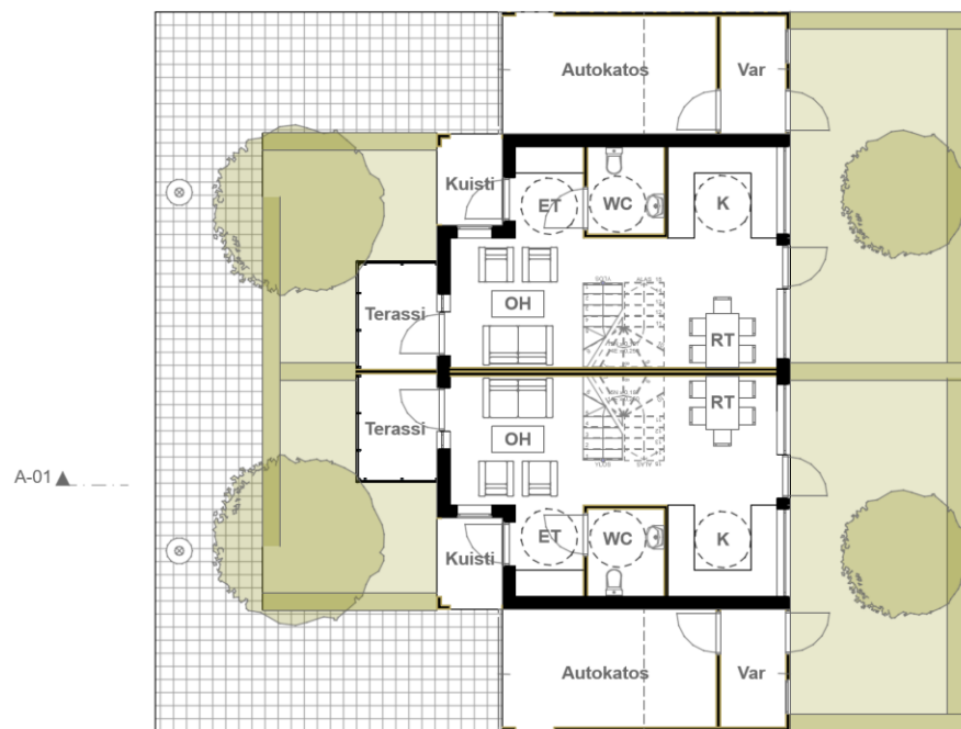
1. våningen plan
