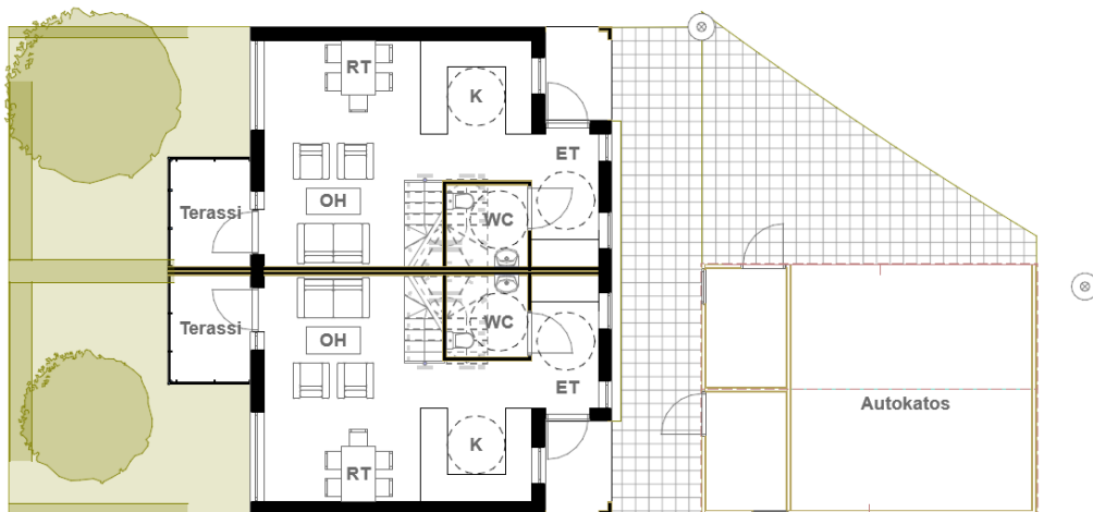
1. krs pohjapiirros
