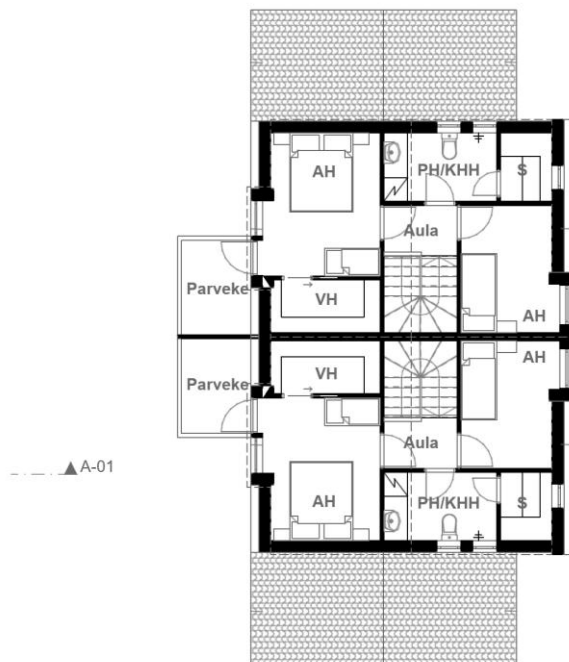
2. krs pohjapiirros
