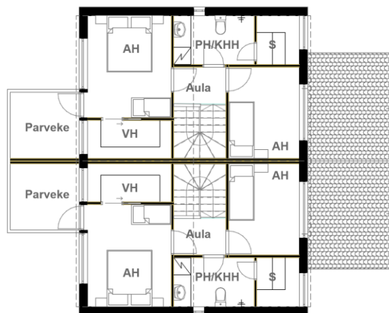
2. krs pohjapiirros
